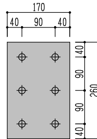
ウェブ 170×260 90ピッチ 3つ穴
