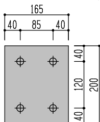
ウェブ 165×200 120ピッチ 2つ穴
