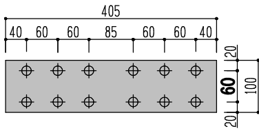
フランジ *60ピッチ 100×405
