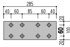
フランジ *60ピッチ 100×285
