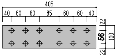
フランジ *56ピッチ 100×405
