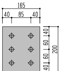
ウェブ 165×200 60ピッチ 3つ穴
