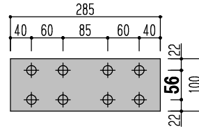
フランジ *56ピッチ 100×285
